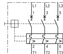
(Принципиальная схема)
